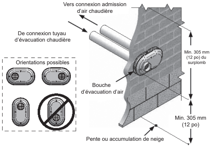
Figure 37. Flux d'entrée et d'évacuation dans les installations à bouche d'extrémité compacte
