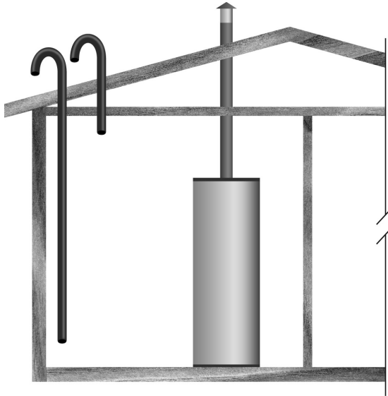
Figure 13. Air extérieur à travers deux conduits verticaux
