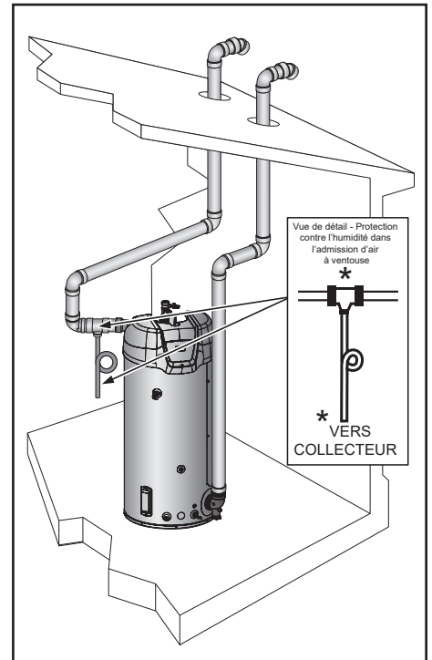
Figure 41. Ventouse verticale
