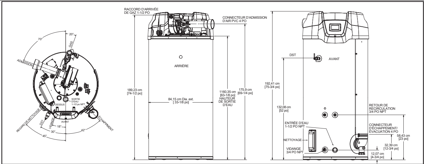
Figure 6. Dimensions de mise en place des conduites
