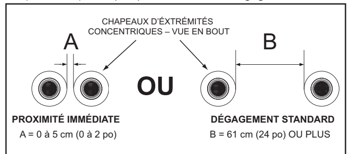
Figure 28. Deux bouches concentriques
