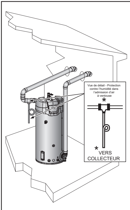
Figure 42. Ventouse horizontale
