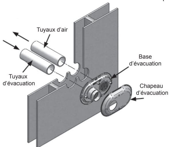
Figure 36. Flux d'entrée et d'évacuation dans les installations à extrémité compacte
