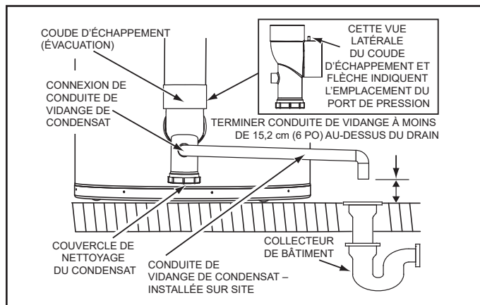
Figure 9. Coude d'échappement/condensat
