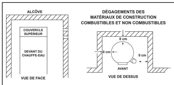
Figure 7. Dégagements
