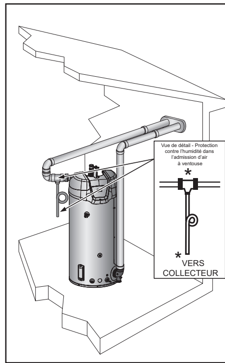
Figure 47. Ventouse compacte horizontale
