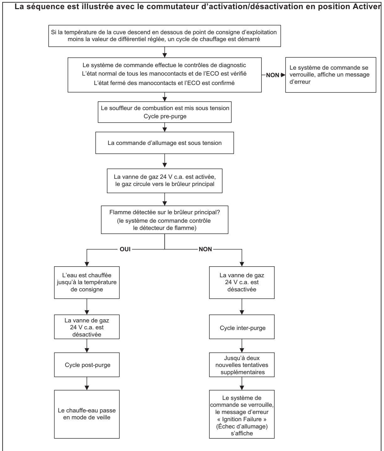
Figure 58. Séquence de fonctionnement
