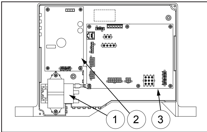
Figure 55. Composants du système de commande
