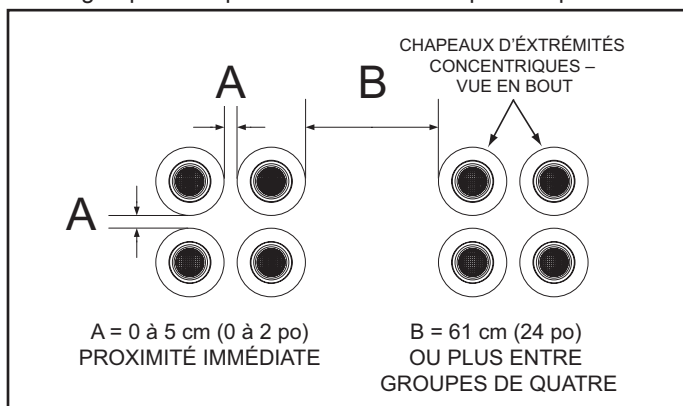
Figure 32. Huit bouches concentriques
