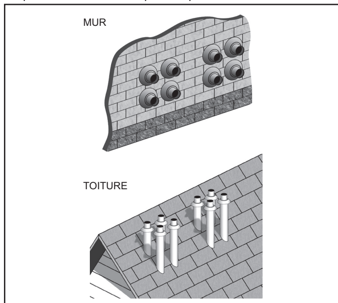
Figure 35. Huit bouches concentriques - Mur et toit
