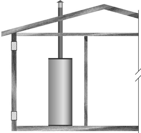
Figure 10. Air extérieur à travers deux ouvertures
