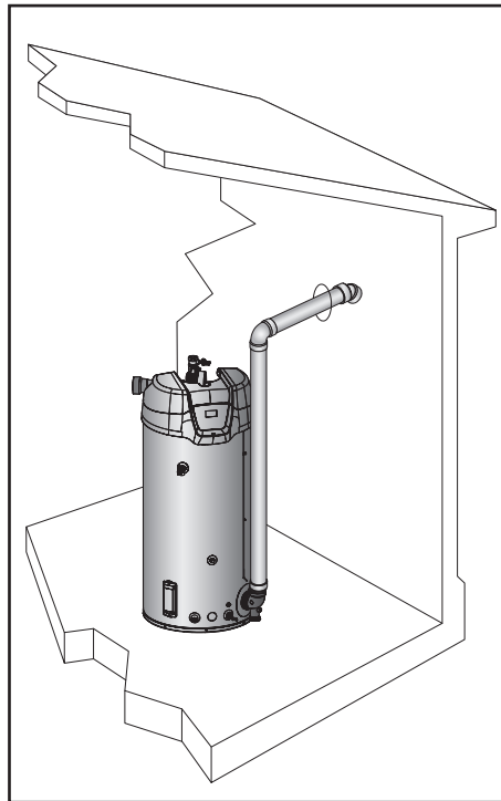
Figure 40. Évacuation mécanique horizontale
