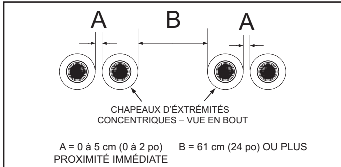
Figure 31. Quatre extrémités concentriques en ligne
