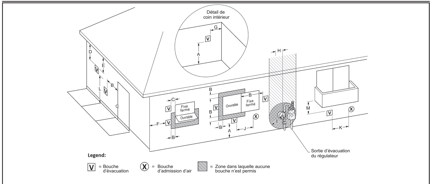
Figure 49. Évacuation autre qu'à ventouse murale utilisant l'air extérieur
