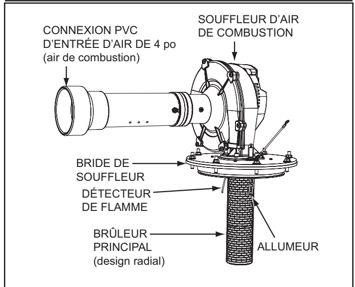
Figure 2. Composants du souffleur/brûleur BTH
