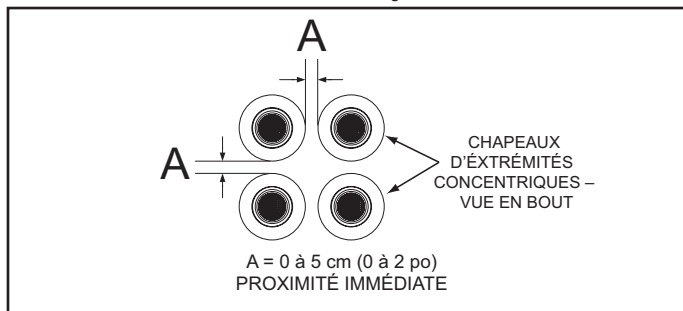
Figure 30. Quatre extrémités concentriques - Proximité immédiate
