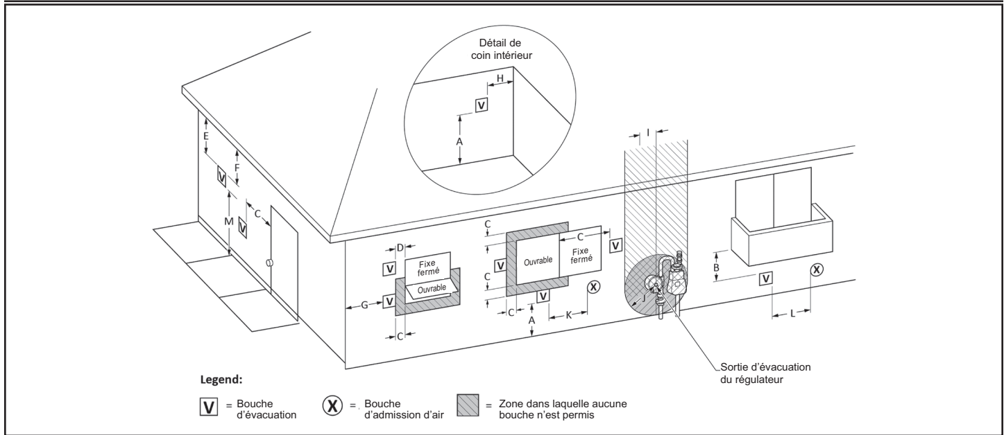
Figure 48. Évacuation à ventouse murale utilisant l'air extérieur
