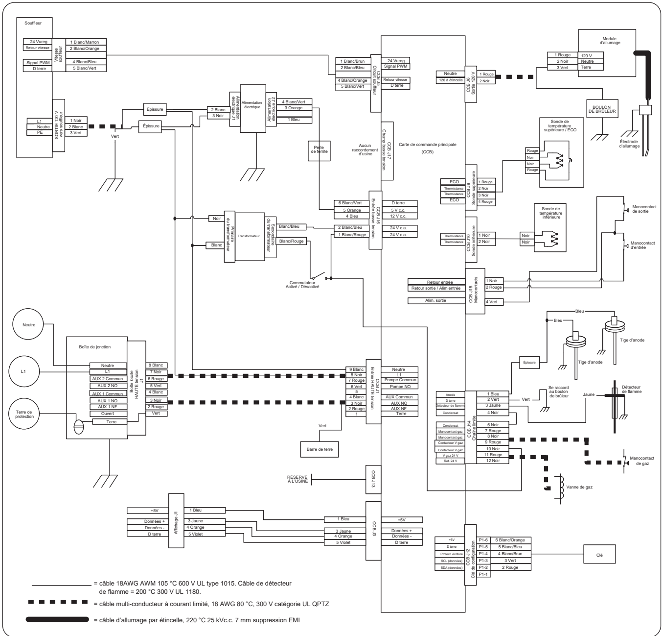
Figure 64. Schéma de câblage
