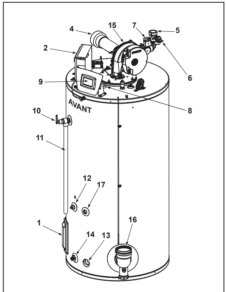
Figure 5. Composants du côté droit
