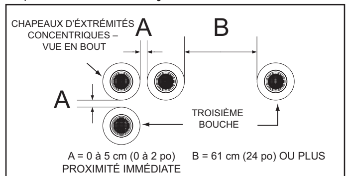
Figure 29. Trois bouches concentriques
