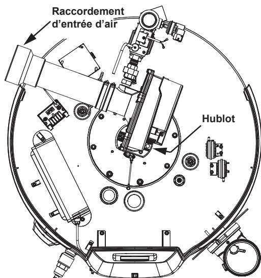
Figure 59. Emplacement du hublot
