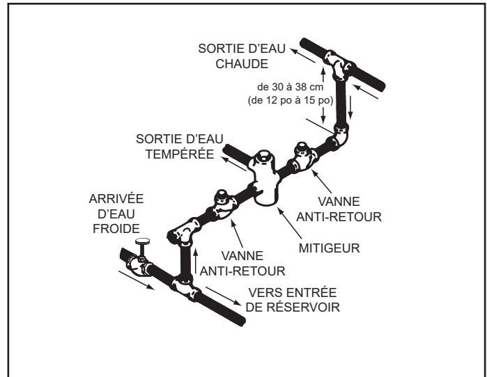
Figure 8. Mitigeur
