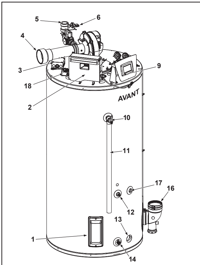
Figure 4. Composants du côté gauche
