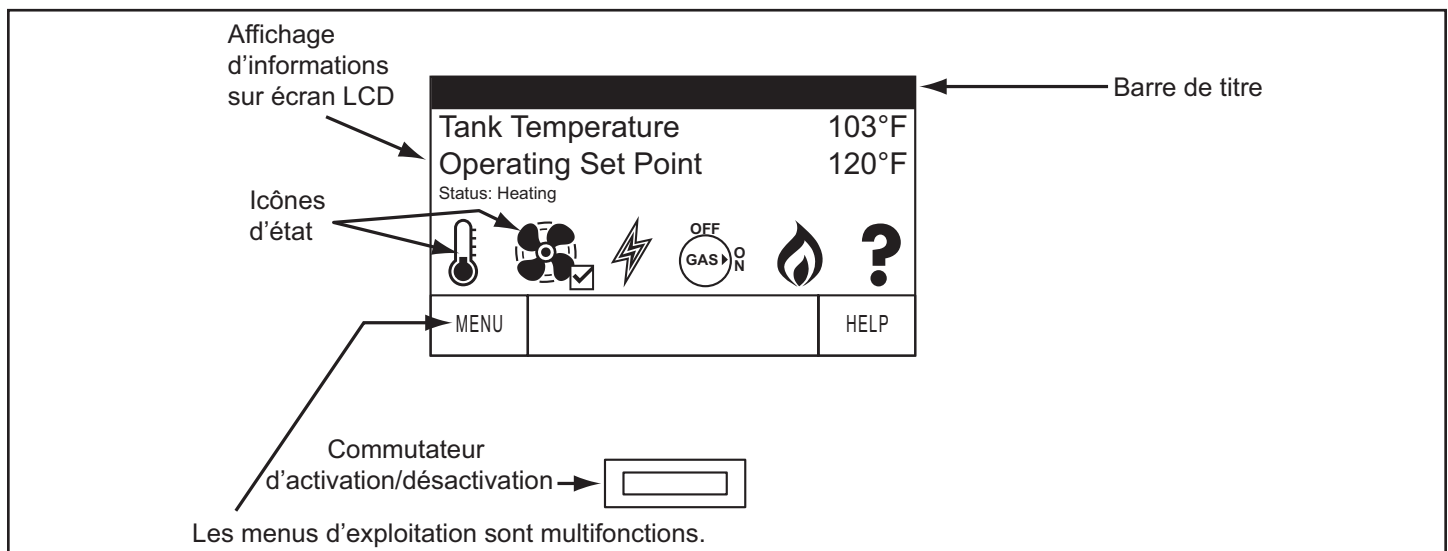
Figure 56. Écran Bureau du module d'interface utilisateur
