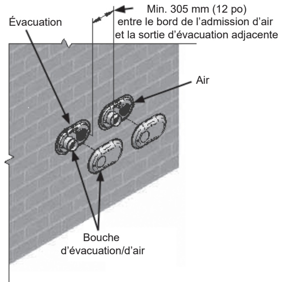
Figure 38. Dégagement entre plusieurs bouches d'extrémité compactes
