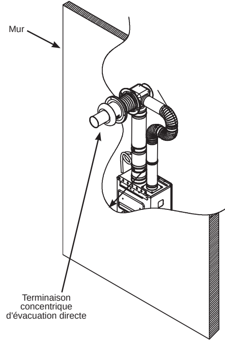
Schéma d'installation horizontale avec terminaison concentrique à évacuation directe
