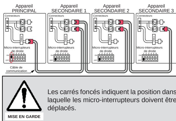
(B) Schéma de base des branchements entre les appareils du système Easy-Link.
