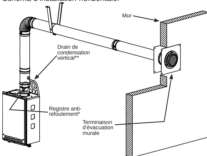
Schéma d'installation horizontale:
