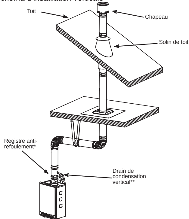
Schéma d'installation verticale
