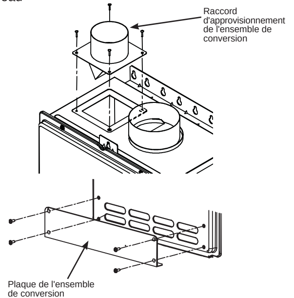
Schéma d'installation de l'ensemble de conversion du chauffe-eau
