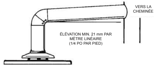
FIGURE 17. PENTE ASCENDANTE MINIMALE DU TUYAU D'ÉVACUATION
