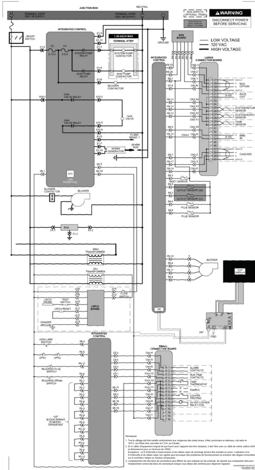
Figure 13-1 Diagrammes en escalier - 120V - Modèles 1250 et 1500
