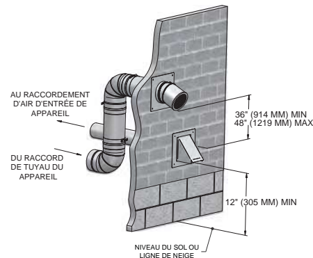
Figure 5-2B Terminaison à paroi latérale en acier inoxydable avec raccords fournis sur place
