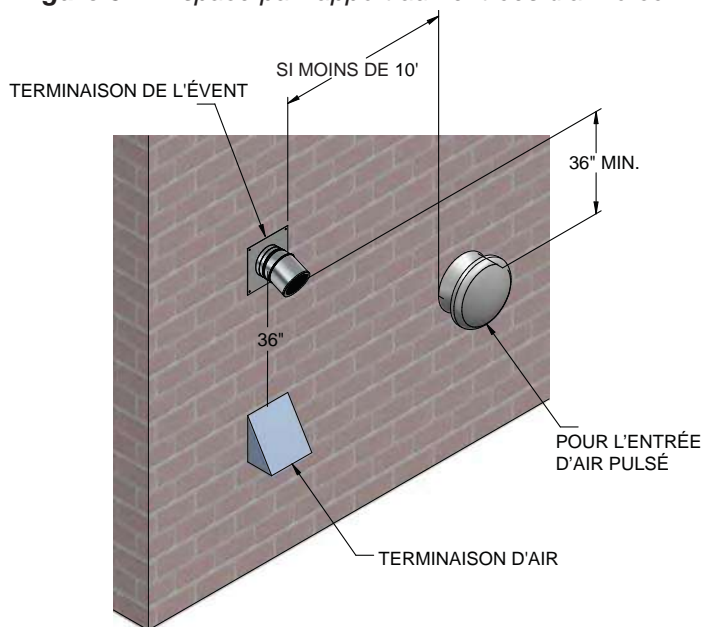
Figure 5-4 Espace par rapport aux entrées d'air forcé
