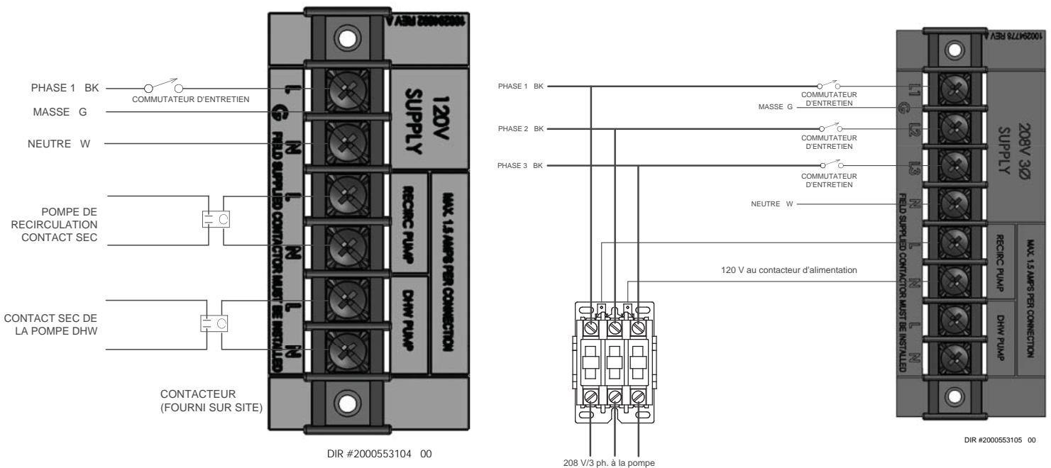
Figure 8-1 Connexions du câblage de tension secteur de la chaudière
