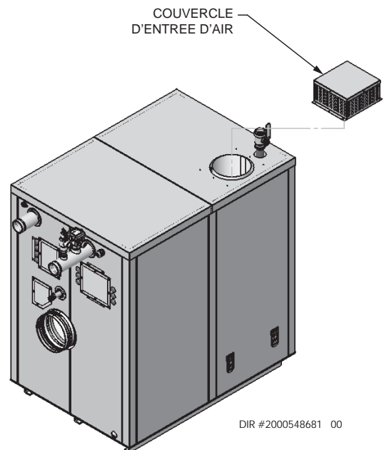
Figure 5-8 Installation d'air ambient
