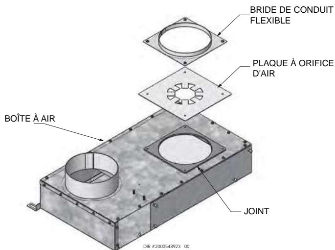
Figure 2-4 Plaque d'orifice d'air d'installation - Modèles 3000 et 4000
