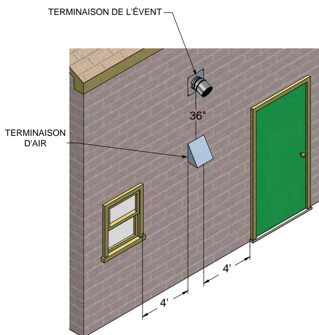
Figure 5-4 Espace par rapport aux entrées d'air forcé
