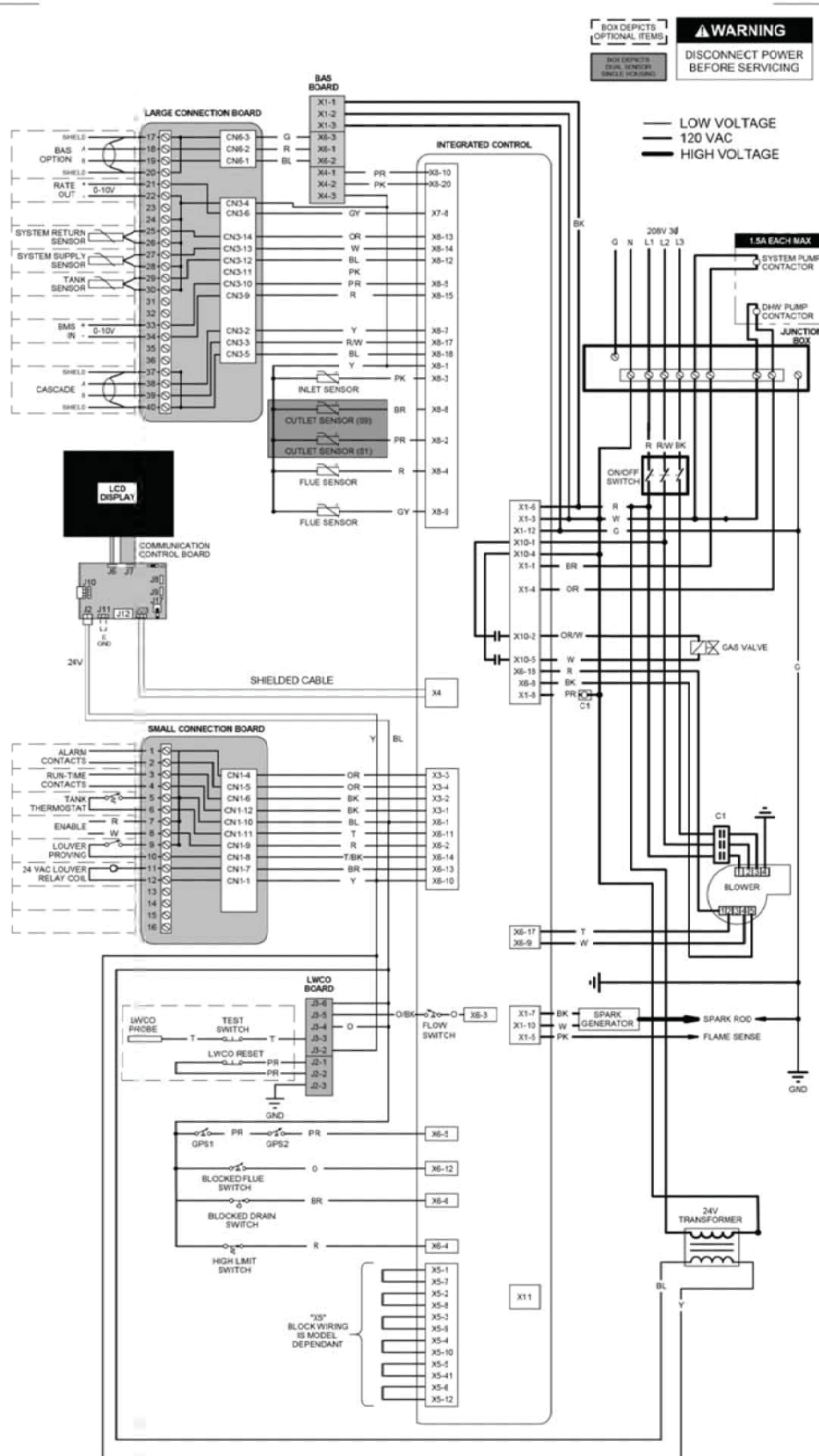
Figure 13-4 Schéma de câblage - 208V - Modèles 2000 et 3000
