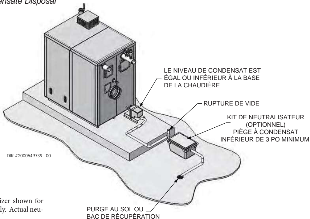
Figure 9-1 Condensate Disposal
