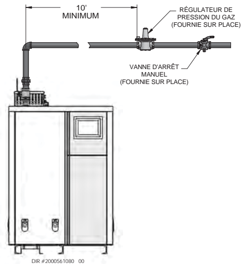
Figure 7-3 Tuyauterie d'alimentation en gaz vers le régulateur
