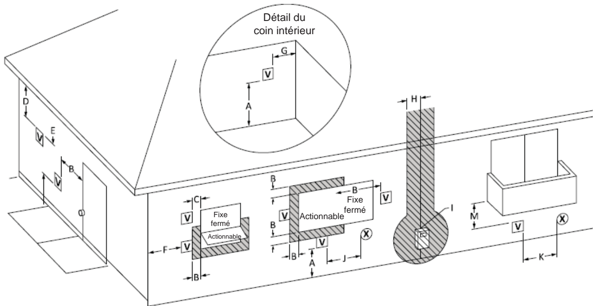
Figure 5-10 Autres que les espaces de terminaison de ventilation directe
