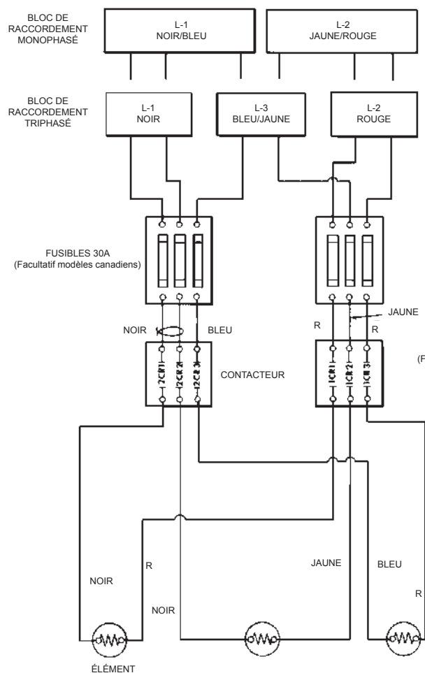
TROIS ÉLÉMENTS - MONOPHASÉ ET TRIPHASÉ
