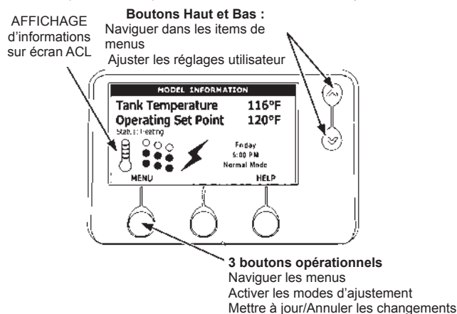
UIM - MODULE D'INTERFACE UTILISATEUR
