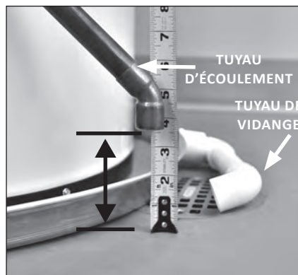
Figure 13 - Le tuyau d'écoulement de la soupape DST doit déboucher à un maximum de 305 mm (12 po) au-dessus d'un avaloir de sol ou à l'extérieur du bâtiment.
