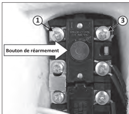
Figure 23 - Bouton du limiteur ECO.
