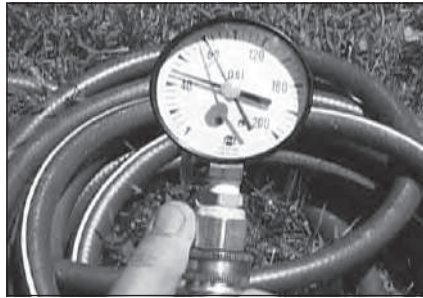
Figure 4 - Utiliser un manomètre à eau pour s'assurer que la pression d'eau n'est pas trop élevée.
