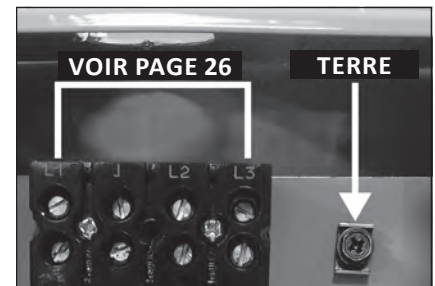
Figure 19 - Raccorder les fils électriques.
