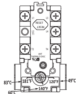
Figure 36 - Thermostats supérieur et inférieur.
