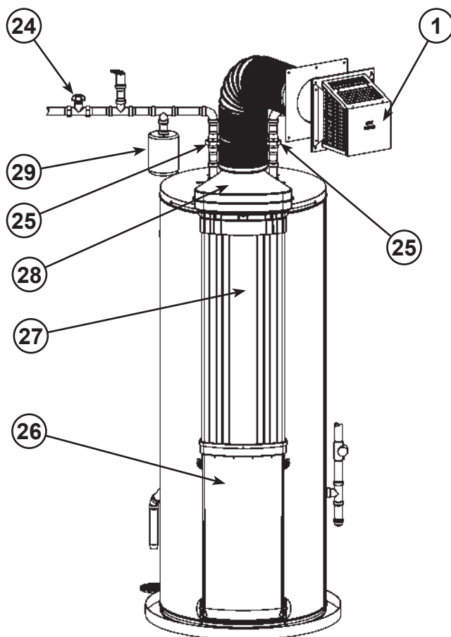
Vue arrière
